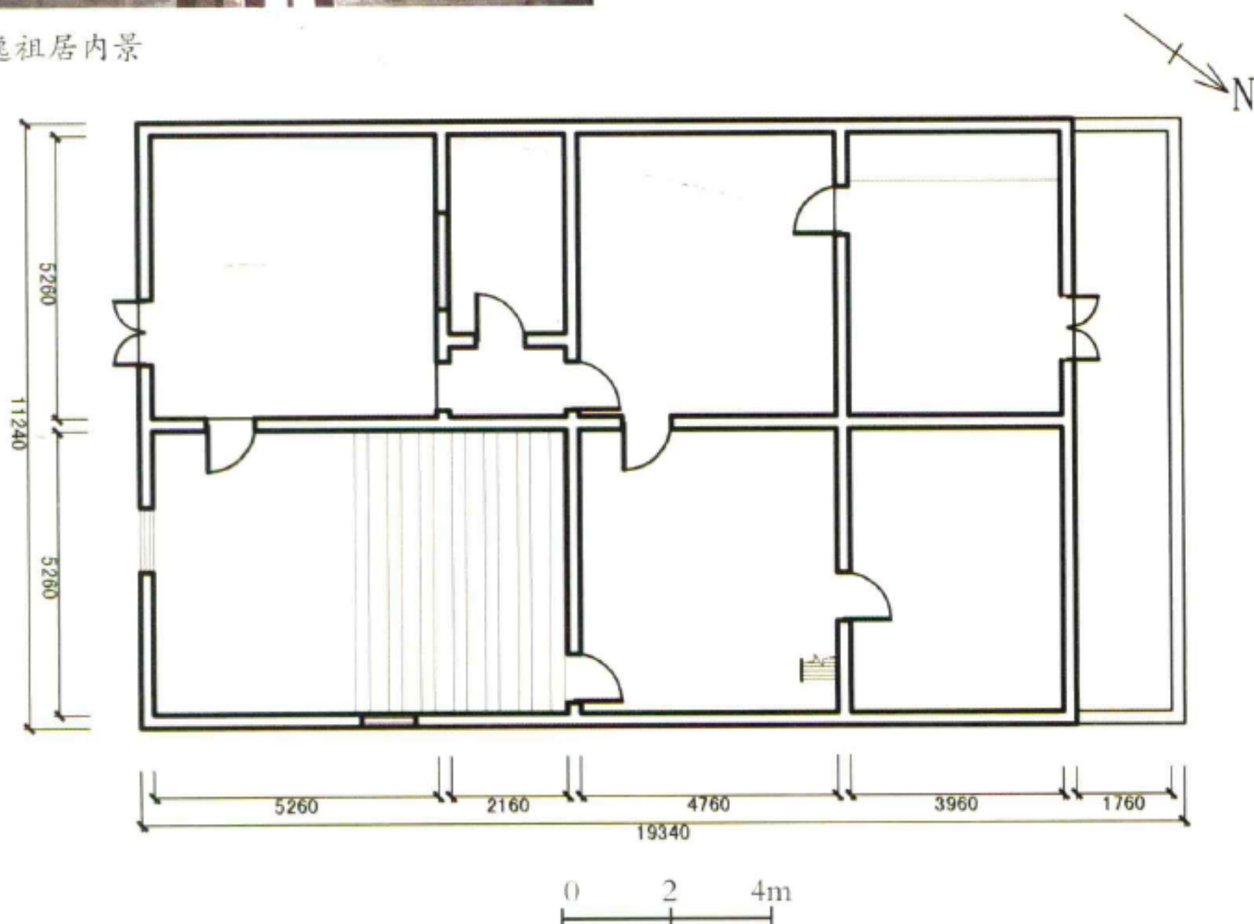
杨仙逸祖居平面示意图
