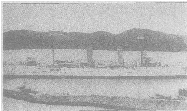
■“海琛”号在德国完工后驶入大沽口时的情景
